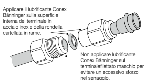
Fig. 2 Raccordo con terminale in acciaio inox e rondella cartellata in rame
