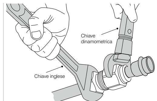
Fig. 3 Serrare la giunzione utilizzando una chiave dinamometrica.
