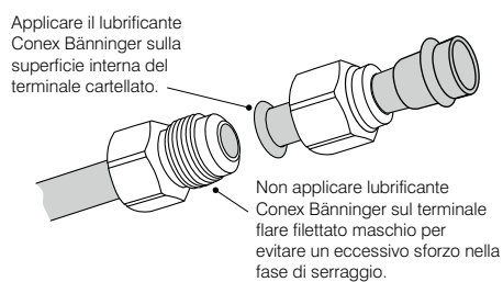
Fig. 1 Raccordo cartellato in rame.
